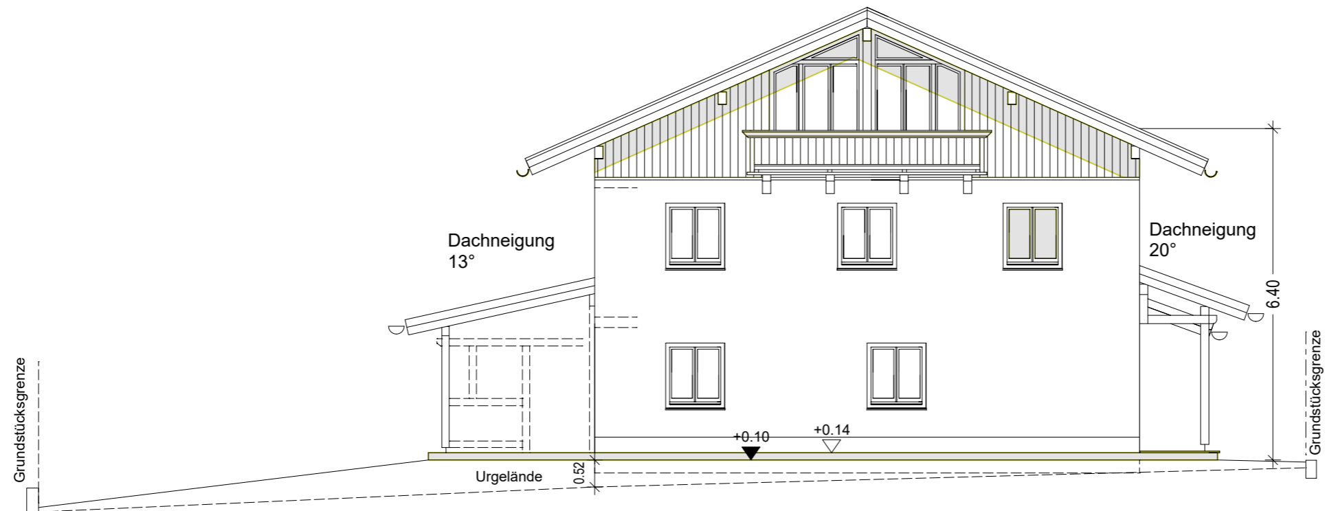
Ansicht - Ost
