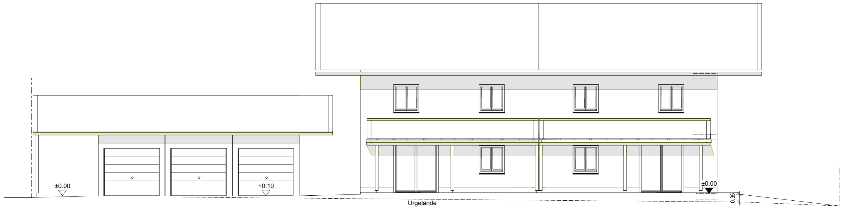
Ansicht - Süd
